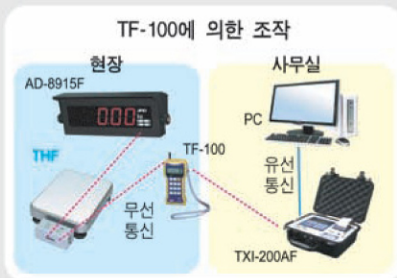
예2) 실시간 데이터 전송
