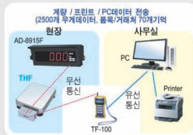
예3) TF-100에서 무게값 기억후 일괄 프린터 및 PC전송
